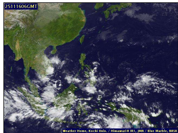
ภาพถ่ายดาวเทียม วันที่ ๑๖ พ.ย. ๒๕๖๘ เวลา ๑๓.๐๐ น.
