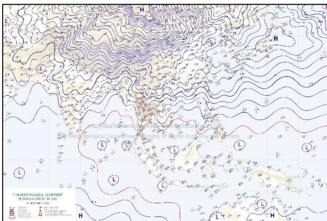
แผนที่อากาศ วันที่ ๑๖ พ.ย. ๒๕๖๘ เวลา ๐๗.๐๐ น.
